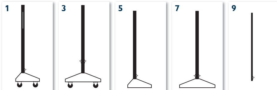
1 RNS Fahrregal, niedrig, 1-seitig bestückbar Mobile rack, low, for single-sided use
