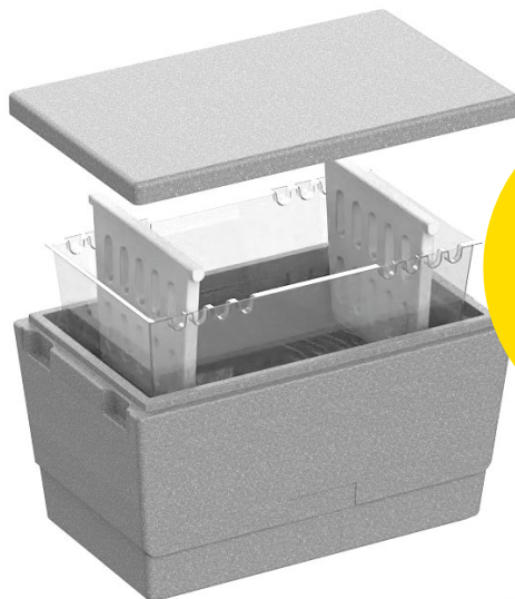
Verstärkung Randgeometrie Reinforced Edge geometry
