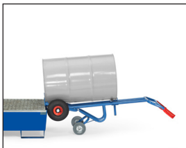
Abstellen eines Fasses auf einer Auffangwanne.
