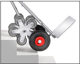
Fünfarmiger Radstern AK1327 | AK1328
