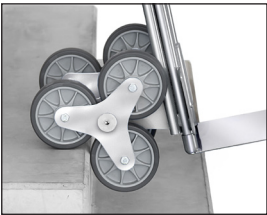
Dreiarmliger Radstern AK1325 | AK1326
