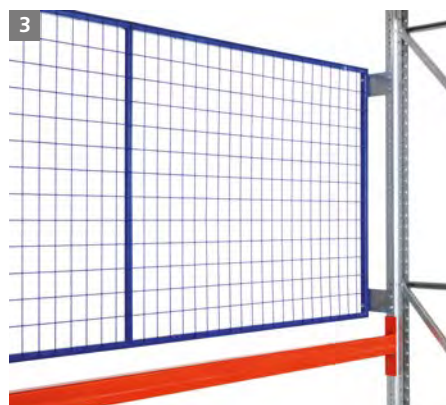
3 Rückwandgitter HEAVY · Oberfläche RAL 5010 enzianblau · ohne Befestigungszubehör
