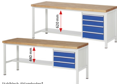
Stahlblech-Ablageboden*
